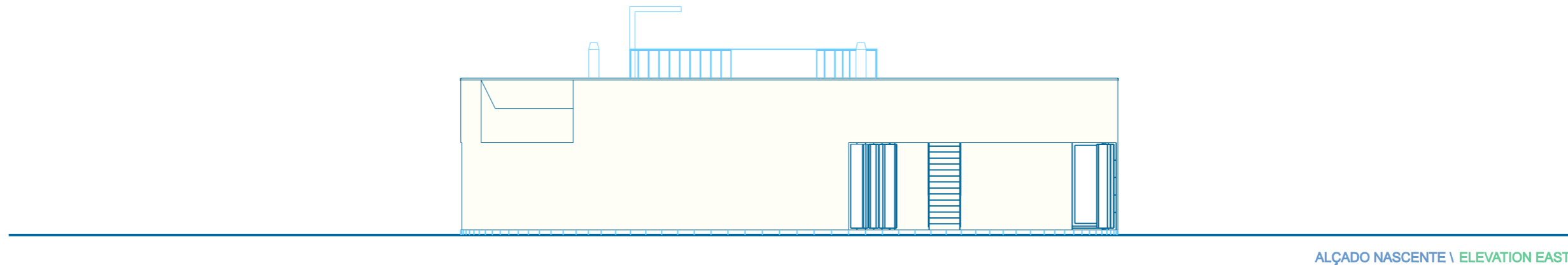
ALÇADO SUL \ ELEVATION SOUTH
